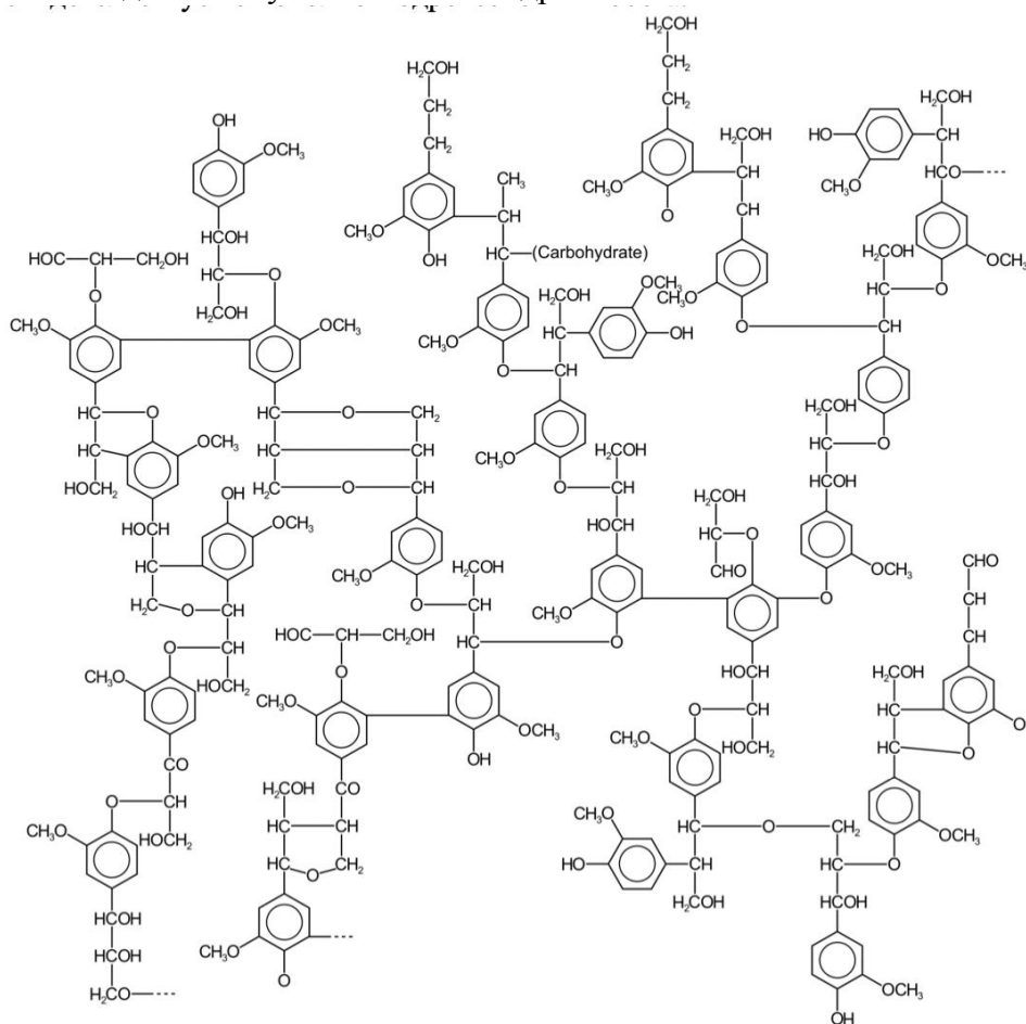
Рис. 1. Структура лигнина
